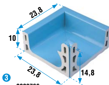
0003766 Canale alto angolo interno 23,8x23,8 / 9 1/2" x9 1/2"
