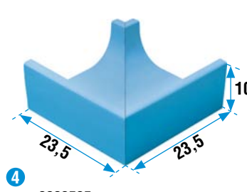
0003535 Canale basso angolo esterno 23,5x23,5 / 9 1/4" x9 1/4"
