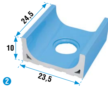
0003533 Canale basso con scarico 24,5x23,5 / 10"x9 1/4"
