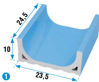
0003532 Canale basso 24,5x23,5 / 10"x9 1/4"
