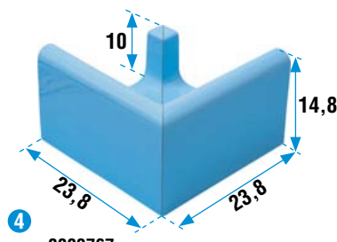
0003767 Canale alto angolo esterno 23,8x23,8 / 9 1/2" x9 1/2"
