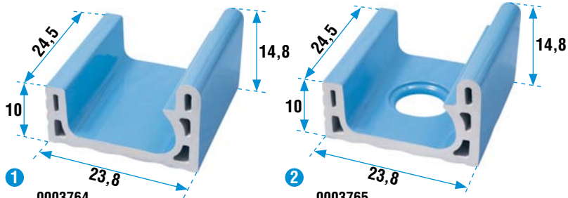
0003764 Canale alto 24,5x23,8 / 10"x9 1/2"
